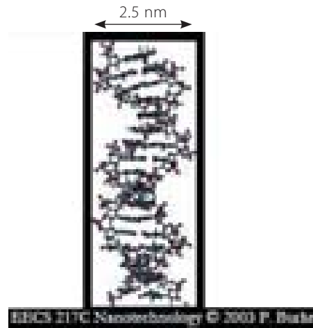
Şekildeki DNA molekülü, 2.5 nanometre enindedir.
