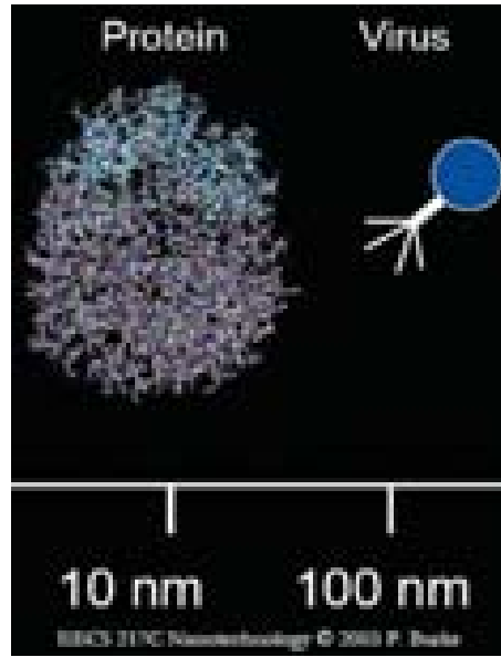
Şekil, tabiatta bulunan protein ve virüslerin boyutlarını göstermektedir.
