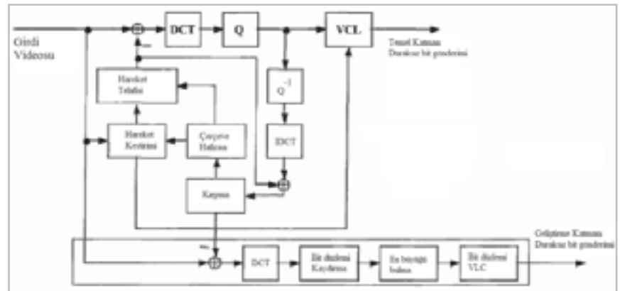
FGS geliştirme katmanının duraksız bit gönderimi herhangi bir noktada piksel başına herhangi bir sayıda bit sonucu dönecek şekilde kod çözme tamamlandıktan sonra kırılabilir. Kod çözücü geliştirilmiş videoyu temel katman ve kırılmış geliştirme katmanı duraksız bit gönderimlerinden tekrar oluşturabilmelidir. Geliştirme katmanı, video kalitesi, alıcının her resim için kod çözdüğü bit sayısı ile orantılıdır. Geniş aralıktaki bit oranını kapsamak için FGS'yi geçici ölçekleme ile birleştirmek gerekir ki sadece resim kalitesi değil, geçici çözünürlük de (çerçeve hızı) ölçeklenebilir olsun [7]. FGS ve katmanlı
