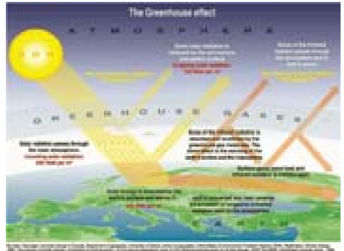
Şekil 1. Sera Etkisi
